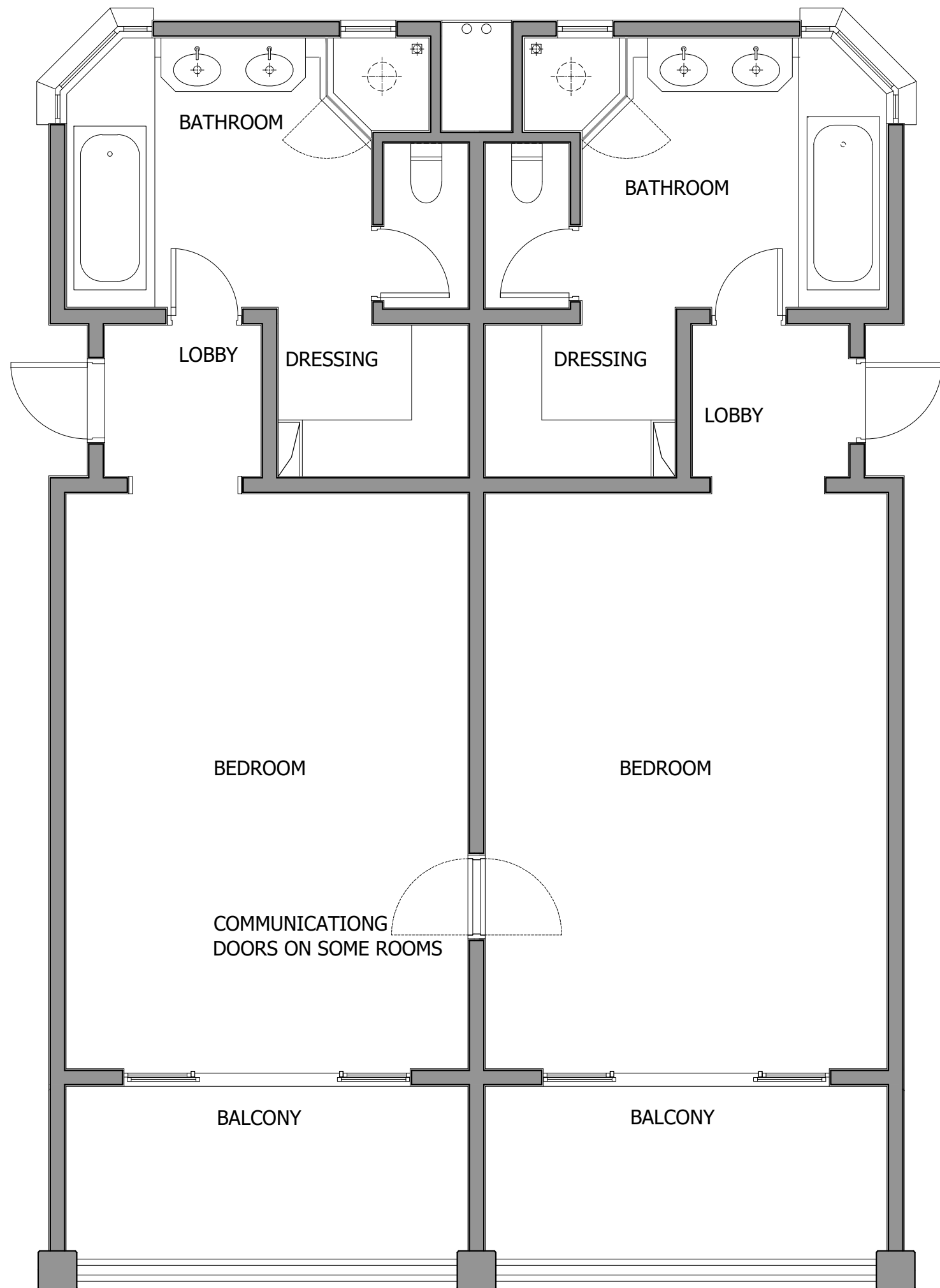
SUPERIOR SUITE PLAN
